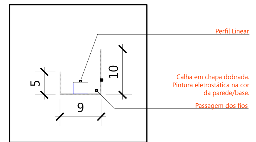
Detalhe B Escala 1/5
